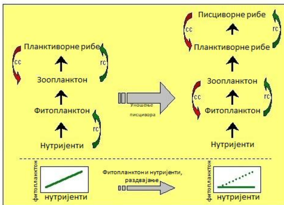
Слика 1. Ланац исхране у воденим екосистемима. На левој страни функционише као систем у три нивоа, а на десној страни, уз претходно додавање писцивора, као систем у четири нивоа. Црвене стрелице означавају контролу потрошача (cc – eng. consumer control ), а зелене стрелице контролу ресурса (rc – eng. resource control ). Прелазак на систем од четири нивоа одваја фитопланктон од нутријената (Drenner & Hambright, 2002).
