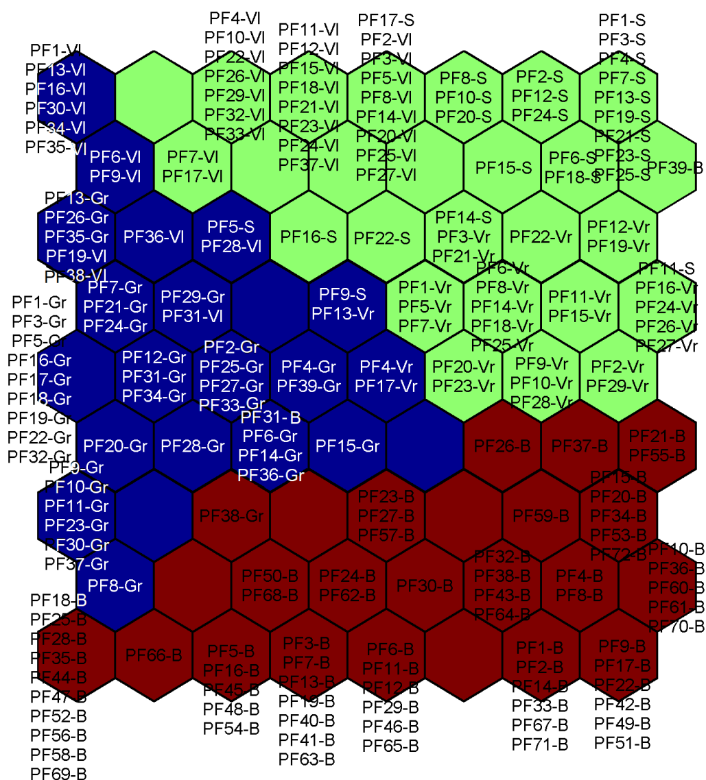
Слика 8. Цревни трактови 203 јединке јувенилног гргеча приказаних кроз 72 COM излазна неурона распоређених у дводимензионалну решетку (8×9). Јединке су представљене скраћеницама које потичу од почетних слова латинског имена врсте и редним бројем јединке, а малом цртом је одвојено велико слово које представља акумулацију из које је јединка узоркована (B - Бован, Gr - Гружа, S - Шумарице, Vr - Врутци, VI - Власина).
