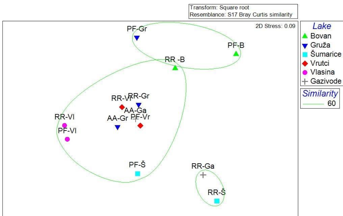
Слика 22. NMDS приказ сличности у исхрани међу јувенилним јединкама сваке врсте из свих истраживаних акумулација. Ординација је заснована на матрици Bray-Curtis коефицијента сличности изведеног из логаритамски трансформисаних ( \log_{10}[x+1] ) %PV вредности категорије плена. Врсте су означене следећим симболима: гргеч PF, бодорка RR и уклија AA.
