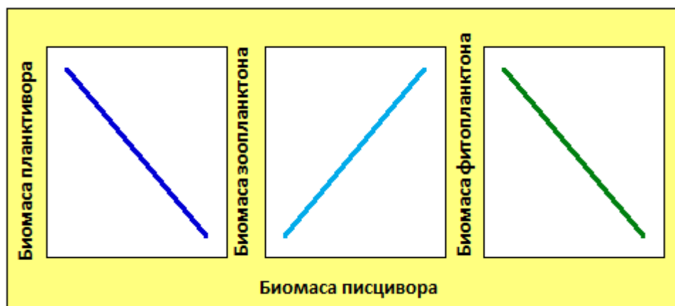
Слика 2. Хипотеза трофичких каскада (модификовано према Carpenter et al., 1985)
