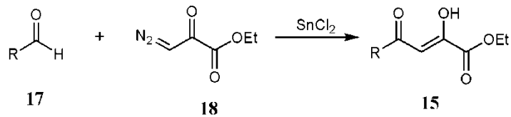
Схема 7. Синтеза ацилпирувата из Diazopyruvate
