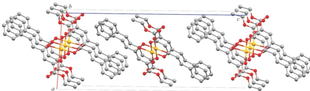
Слика 54. MERCURY 215 приказ кристалног паковања једињења 4Б.
