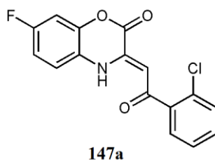
Слика 43. Структура једињења 147a
