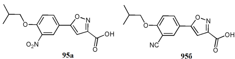
Слика 28. Структуре једињења 95a и 95b
