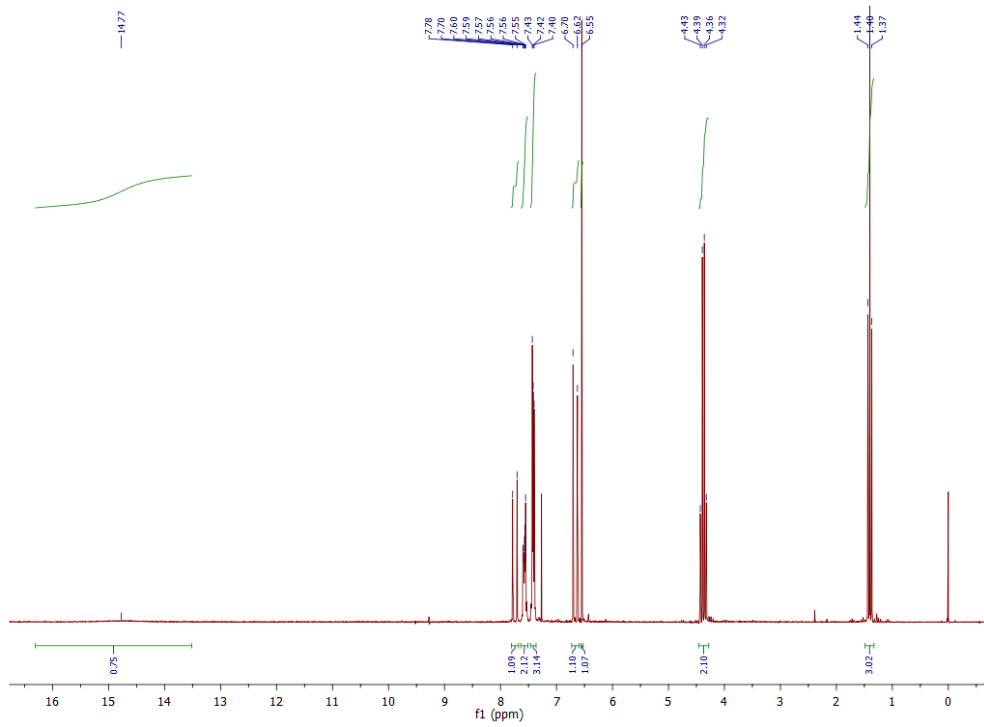
Слика ПЗ. ^1\text{H} NMR спектар једињења 2B
