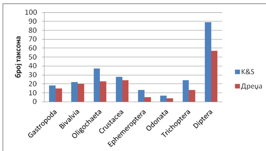
Слика 25. Број таксона унутар најзаступљенијих група макробескичмењака прикупљених К&S методом и дрецом (JDS 3)
