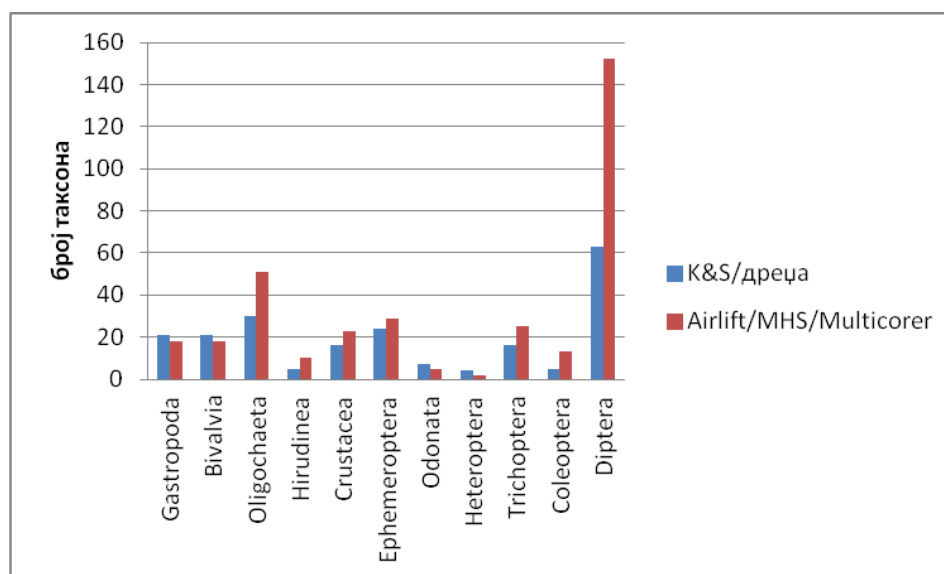
Слика 22. Број таксона унутар најзаступљенијих група макробескичмењака прикупљених K&S/дреца и Air-lift/MHS/Multicorer методама (JDS 2)
